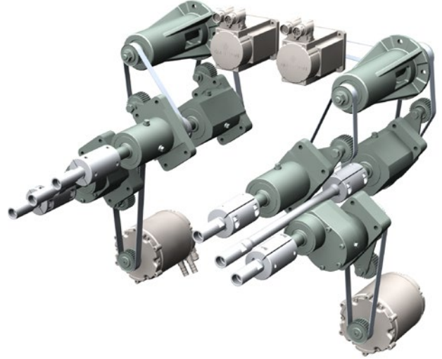
Frekans kontrollü motorlara sahip çekim sistemi tahriki FLEXIdraft
