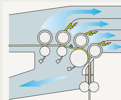
Esquema da aspiração melhorada
