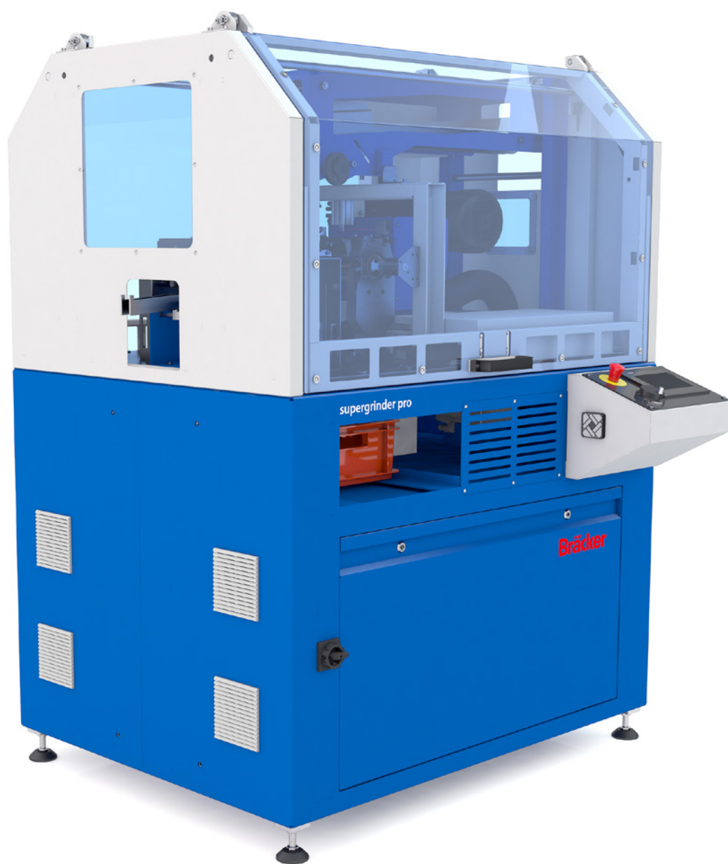
图1：独特的设计使升级版超级磨皮辊机具有更低的能耗、更少的备件、更低的故障风险和更高的产量。
