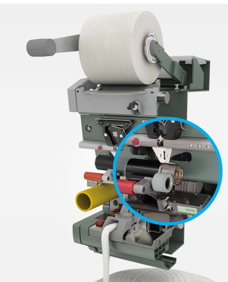
AMIspin-Pro с одним двигателем привода выпуска
