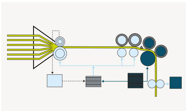
齿轮箱的功能是调节并条机条子重量
